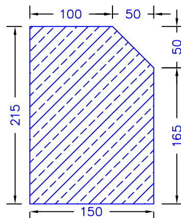
Plinth Section
