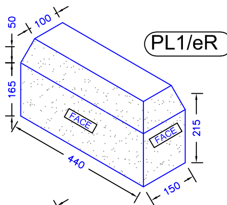
Plinth Section
